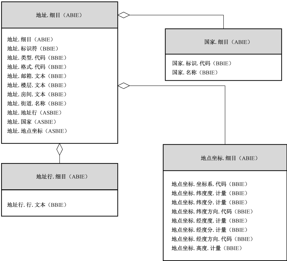
图 1 关联业务信息实体关系结构示例
